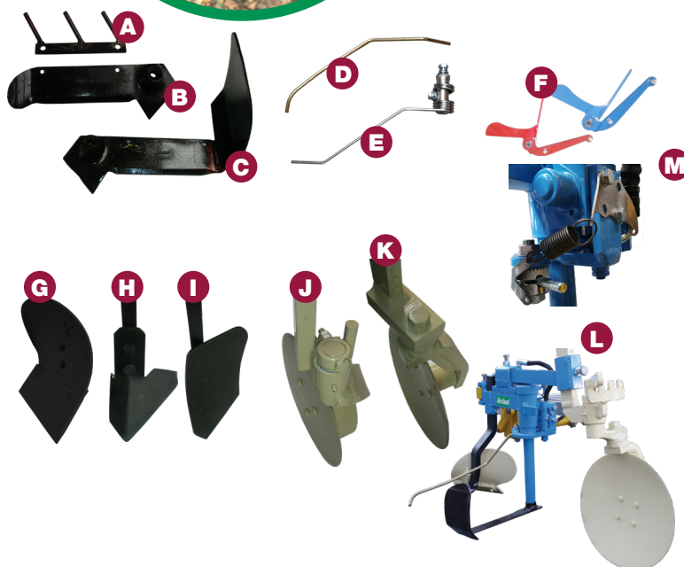
MONTAGE SUR TRACTEUR INTER-LIGNES
